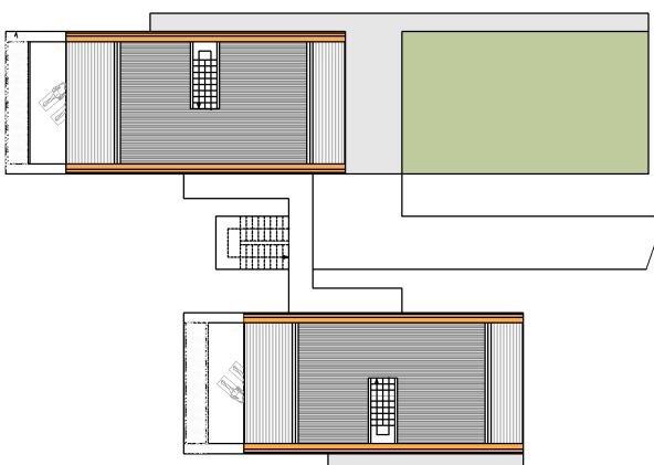
PIANTA PIANO SOTTOTETTO
