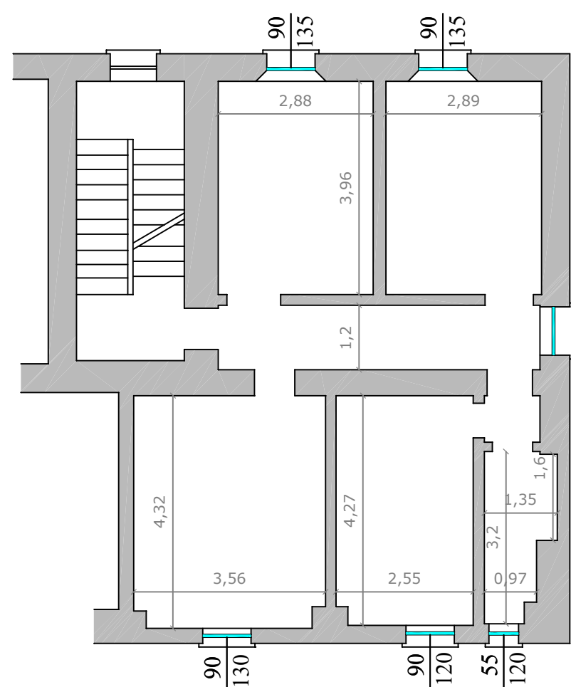
PIANO SECONDO stato di fatto
