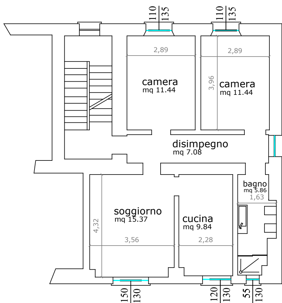
PIANO SECONDO progetto
